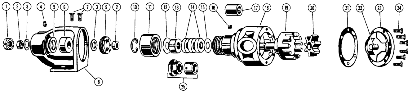
FIGURE 3 VUE ECLATEE SERIES 724 ET 4724 VUE COUPEE SERIE 4724
