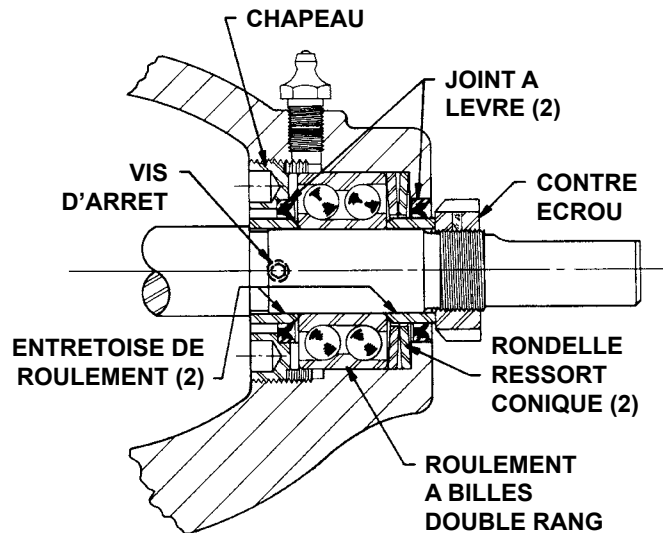
FIGURE 7 VUE COUPEE ROULEMENT DE BUTEE
