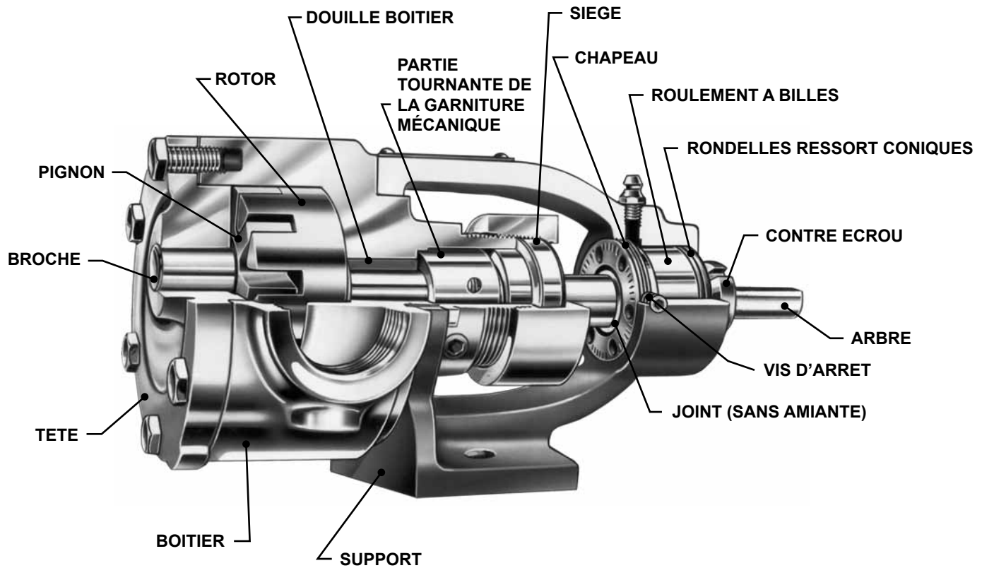
FIGURE 2 – VUE COUPEE SERIE 4724
