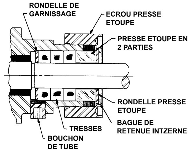
FIGURE 4 VUE COUPEE D'UNE ETANCHEITE A TRESSSES (SERIE 724)
